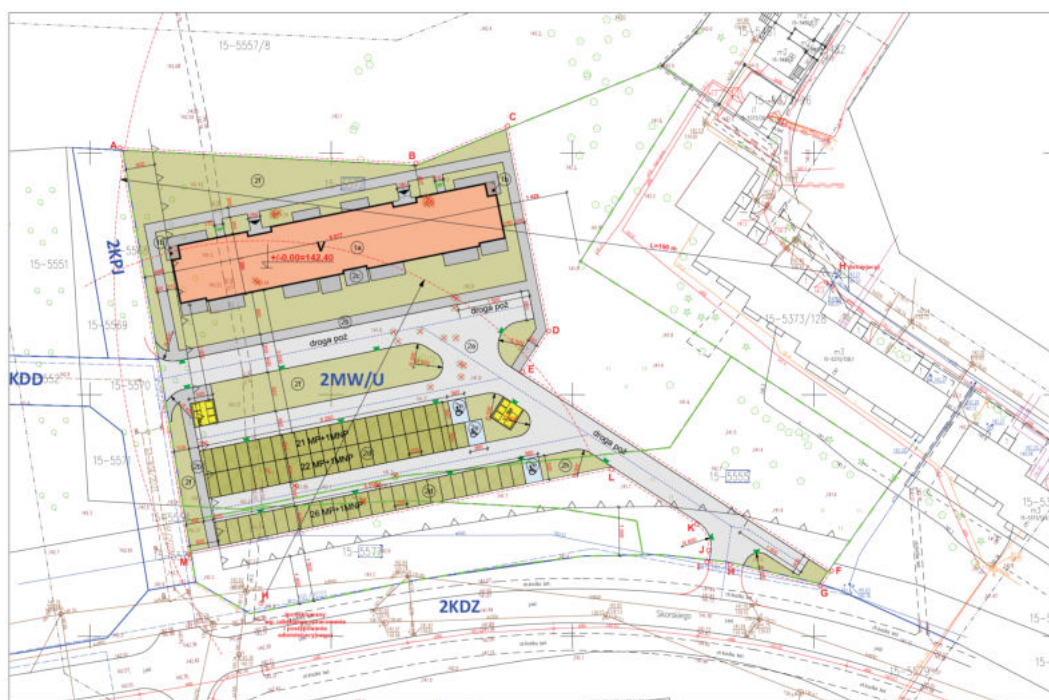
Projekt zagospodarowania terenu
